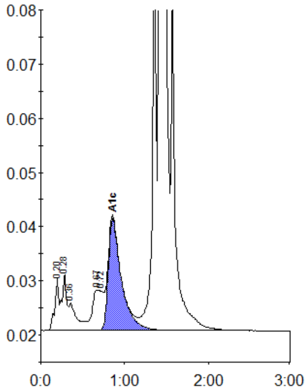
Peak table - ID: 10445397
